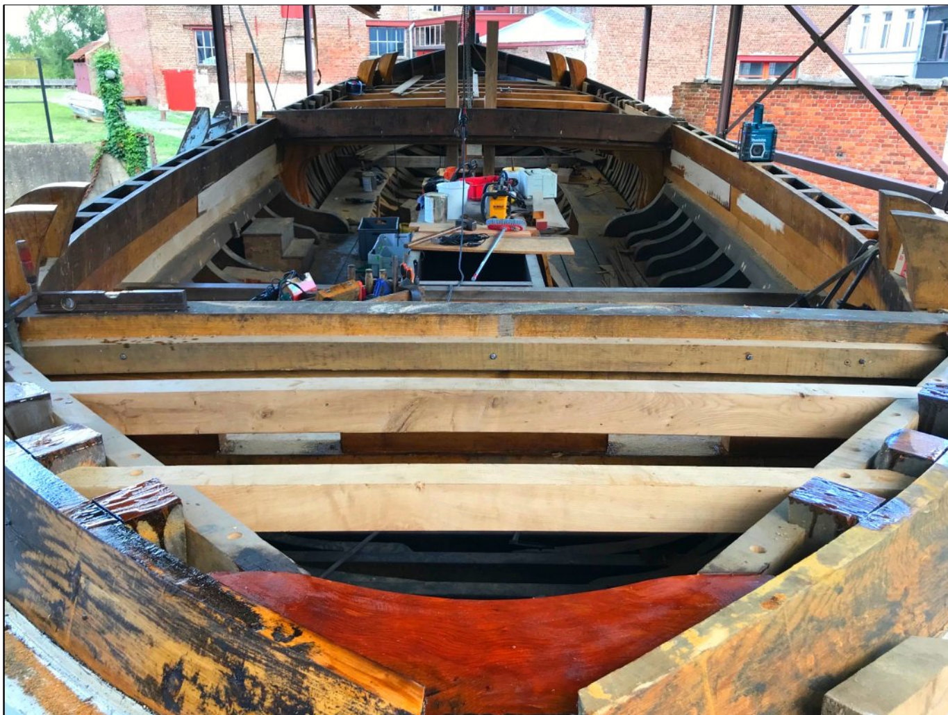
Achterdek balken
