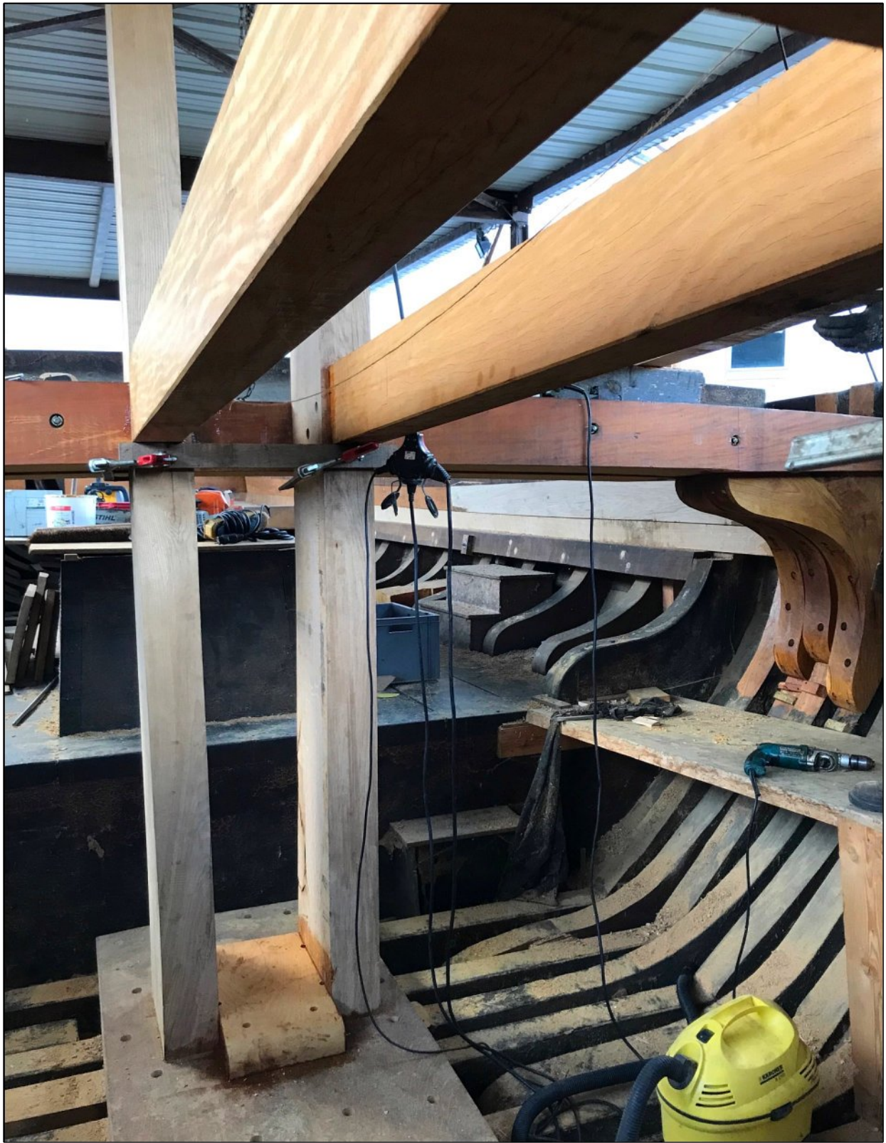
Mastkoker met steunbalken
